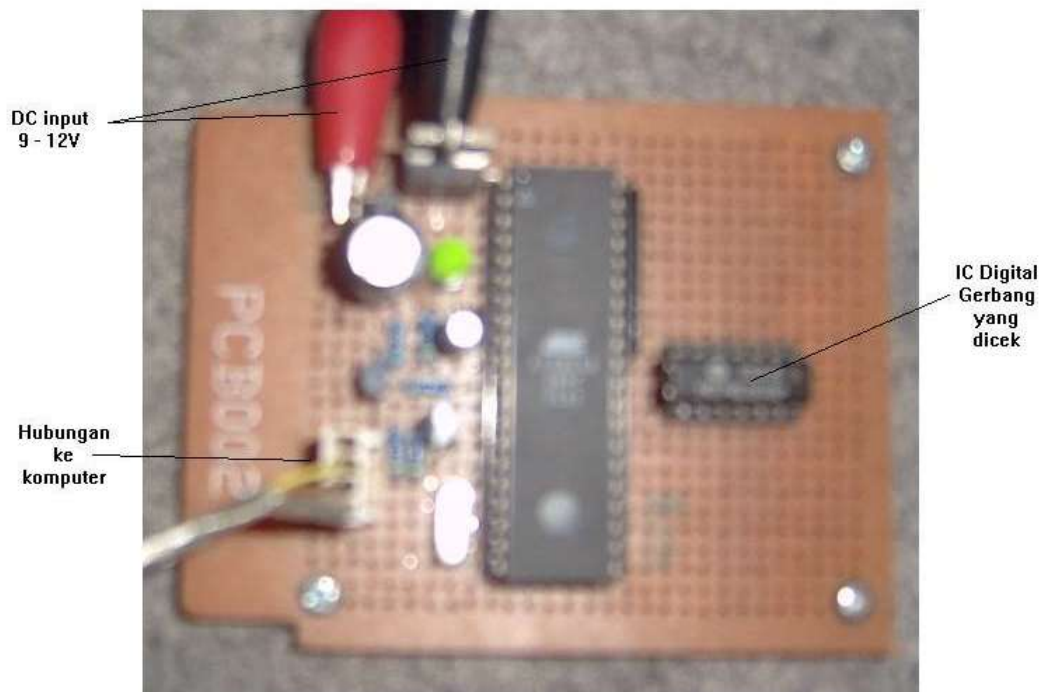
Gambar 3. Modul pendeteksi kerusakan IC Digital Gerbang
