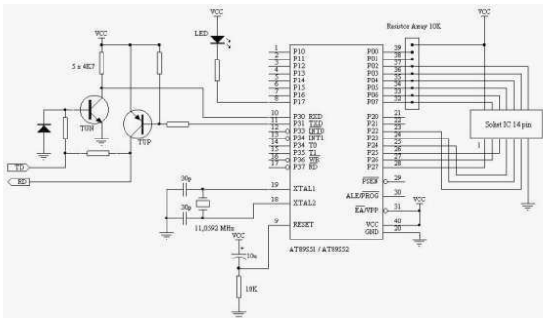
Gambar 2. Skema rangkaian pendeteksi kerusakan IC Digital Gerbang
