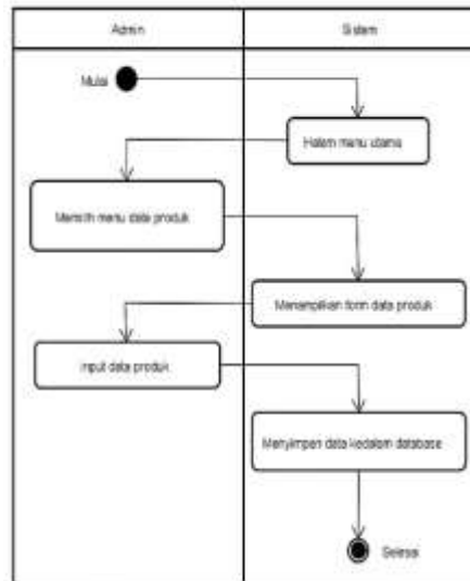
Gambar 11. Diagram Aktivitas Untuk Input Produk
