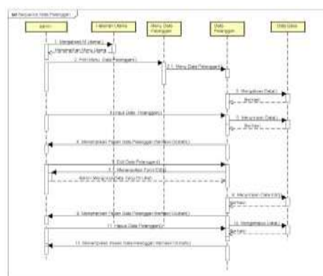
Gambar 7. Diagram Sekuen untuk Menu Pelanggan
