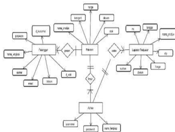
Gambar 1. Diagram Toko Baju Azzahra
