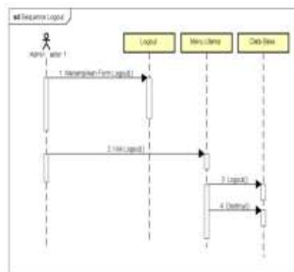
Gambar 5. Diagram Sekuen Logout
