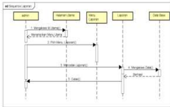
Gambar 8. Diagram Sekuen untuk Menu Laporan
