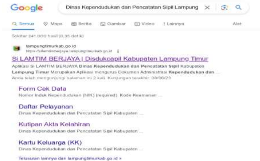
Gambar 2. Menu Login
