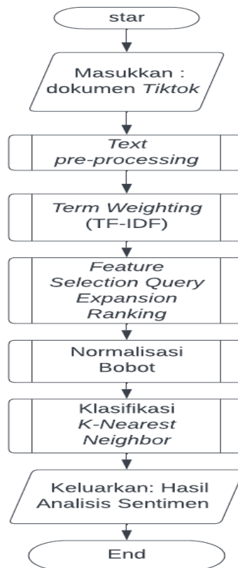
Gambar 1. Diagram Alir Proses Sistem
