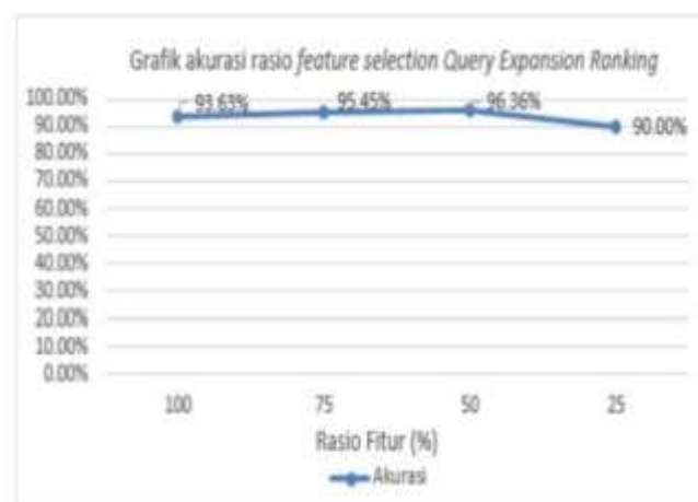
Gambar 3. Grafik Pengujian rasio feature selection
