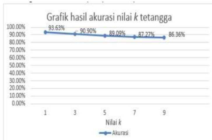
Gambar 2. Pengujian Variasi Nilai k Pada Klasifikasi K-Nearest Neighbor
