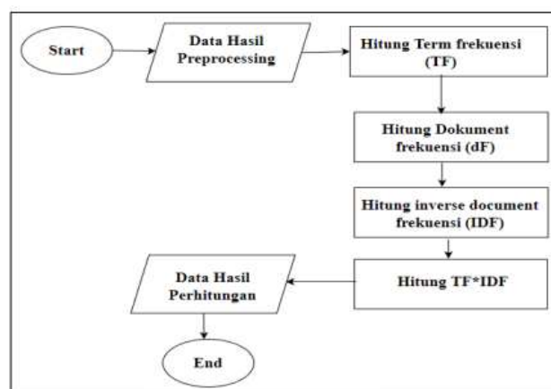
Gambar 2. Pembobotan TF-IDF
